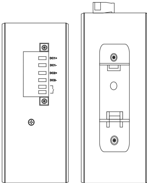
顶视图
