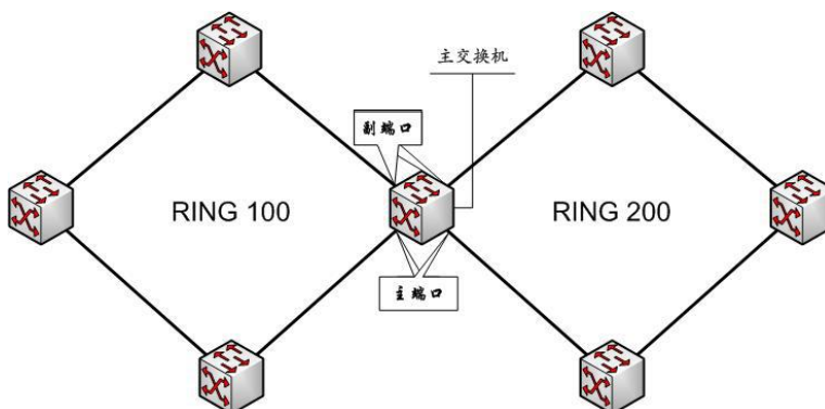
图22.3 相切在主节点的相切环
