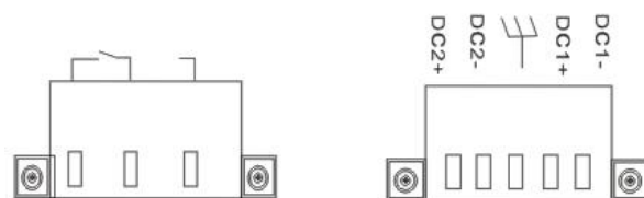
(1): 继电报警接口 (FAIL SAFE) (2): 电源接口
