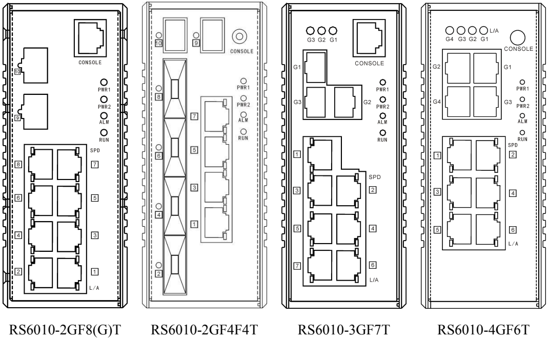
图 1. 1 RS6010 千百兆系列工业以太网交换机前面板示意图
