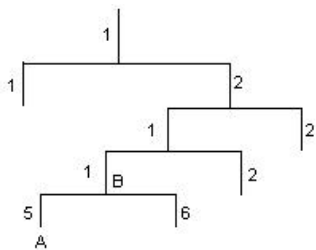
图 15.1 MIB 树结构
