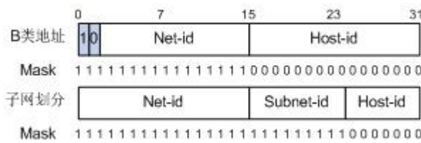
图 6-2 子网掩码
