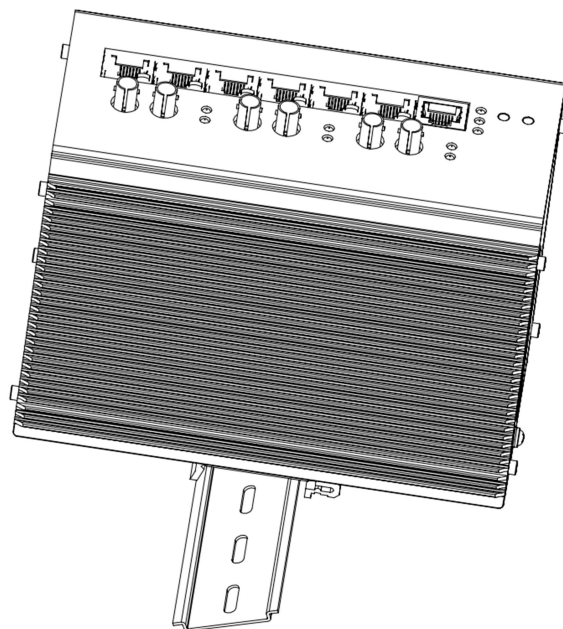
图 2.3 拆除交换机
