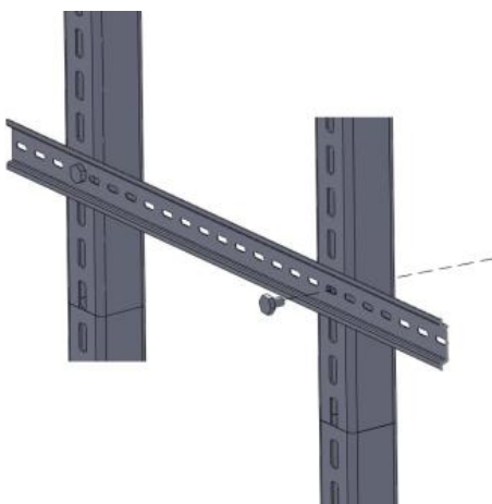
图 2.1 安装导轨
