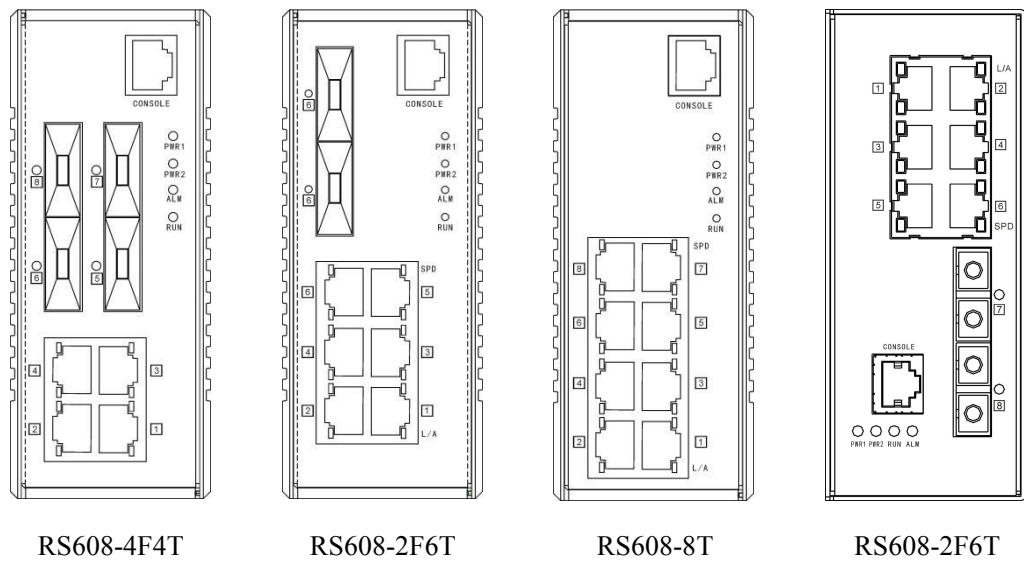
图 1.1 RS608 百兆系列工业以太网交换机前面板示意图
