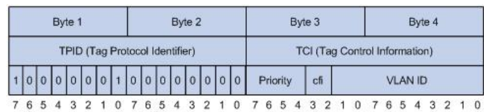
图 11.3 802.1Q 标签头
