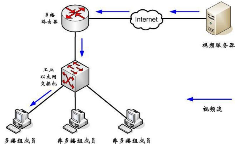
图 5.2 IGMP 对比图
