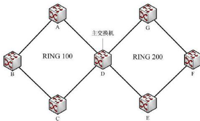
图 5.12 相切于主交换机的相切环
