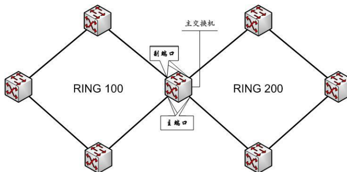
图 5.8 相切在主节点的相切环
