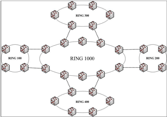
图 5.15 相交环
