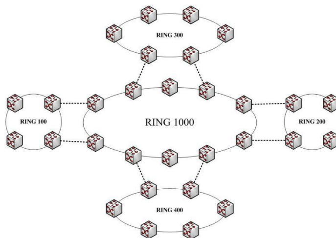
图 5.10 耦合环
