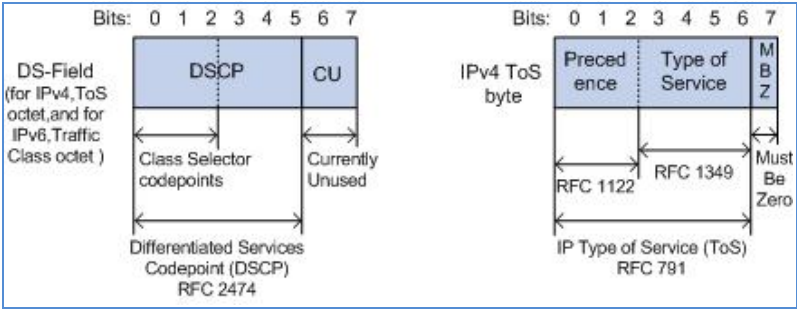
图 5. 5 DS 域和 ToS 字节
