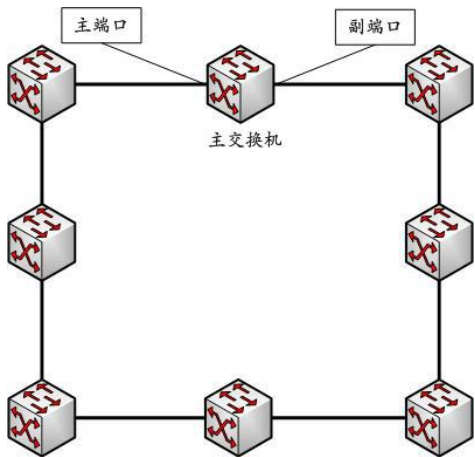
图 5.6 单环
