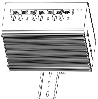
图 2-2 安装交换机
