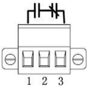
图 2-6 告警端子
